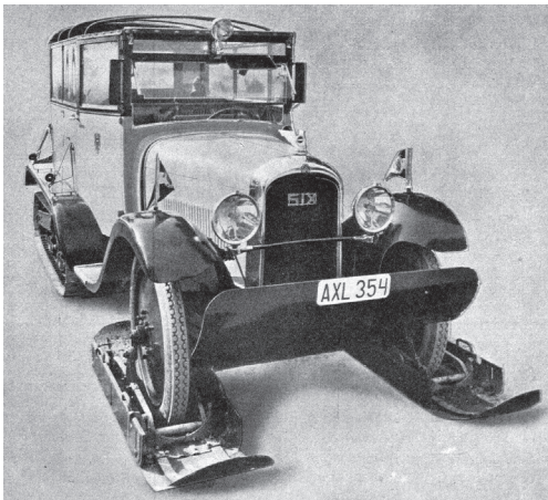
◀ Ein Kégresse-Autobus der österreichischen Postverwaltung
