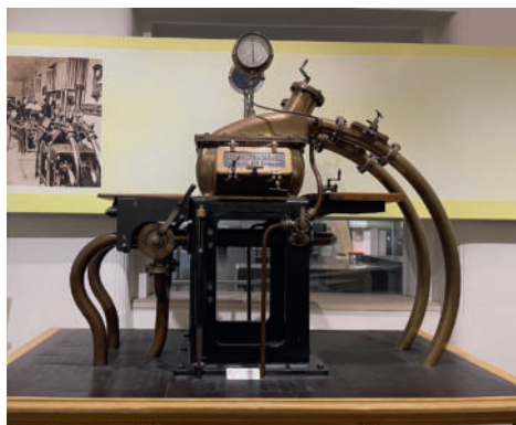
▲ Mittelstation einer Rohrpostanlage, Technisches Museum Wien
